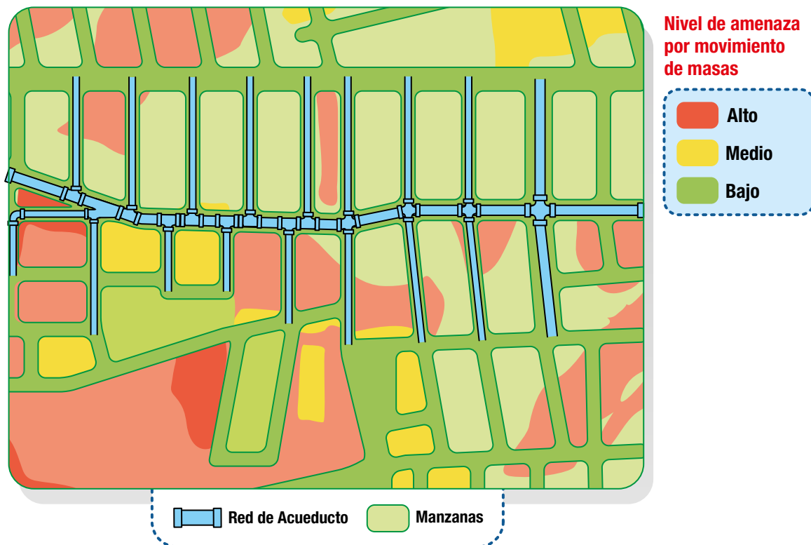
Figura 11. Mapa de superposición de infraestructura sobre amenazas
